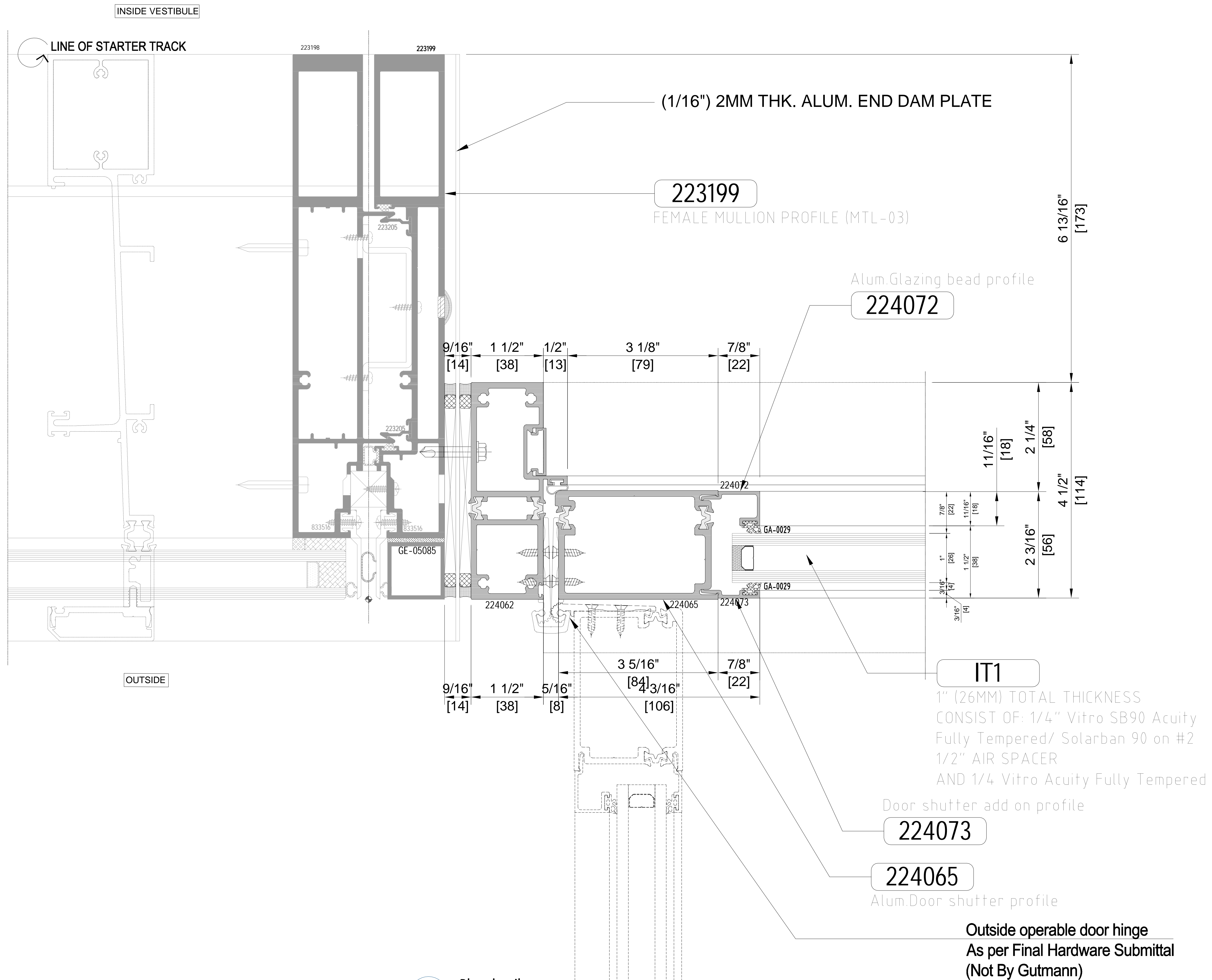
01 Plan detail D-303 Scale: 1:1
